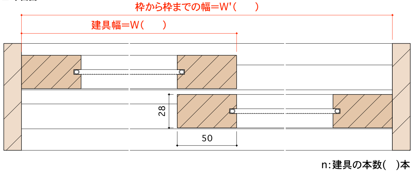
□ 平面図
