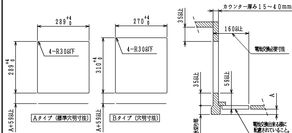
ワークトップ穴開け寸法
