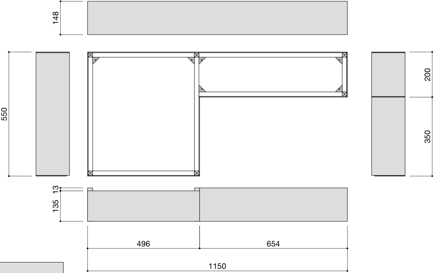
W450食洗機＋シンク用(W1150)配管隠し
