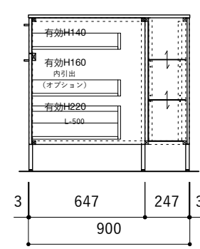
断面図
