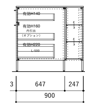
断面図
