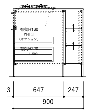
断面図
