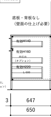
断面図
