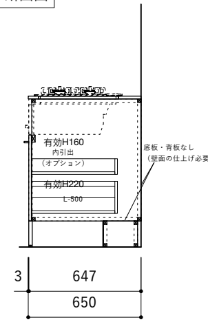
断面図
