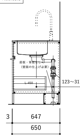
断面図
