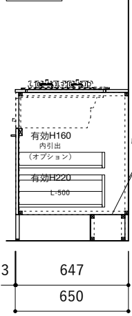
断面図
