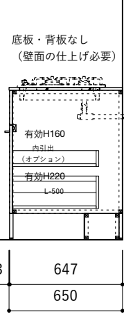
断面図
