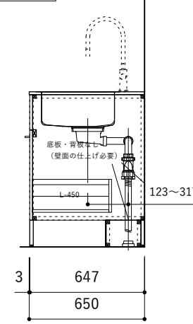
断面図
