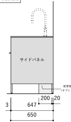
側面図
