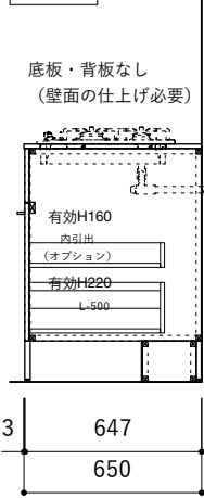
断面図
