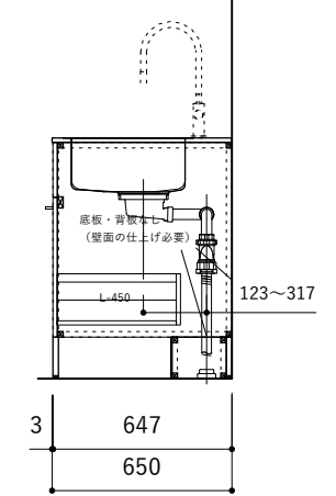
断面図
