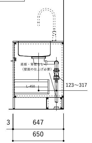
断面図
