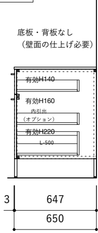
断面図
