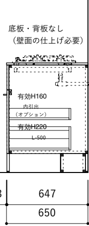
断面図
