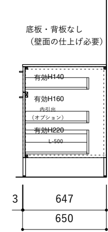
断面図
