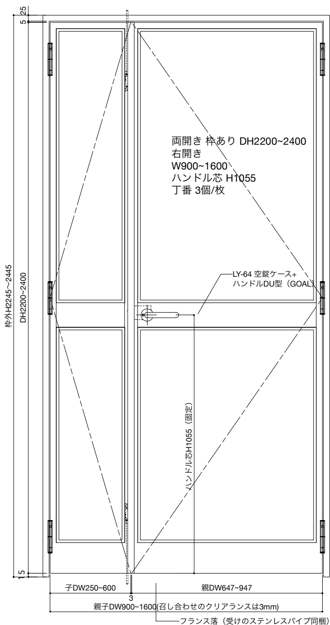
扉表 立面図 S=1:10
