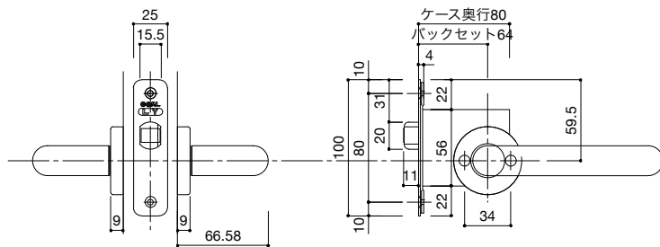
ハンドル詳細図 1/5
