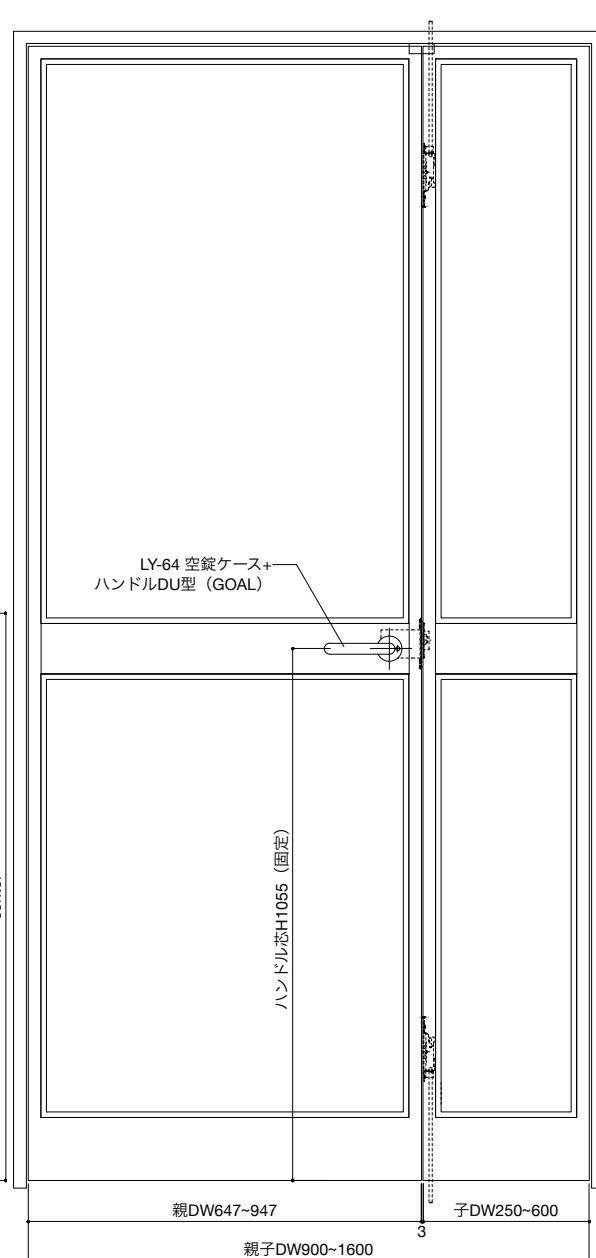
扉裏 立面図 S=1:10
