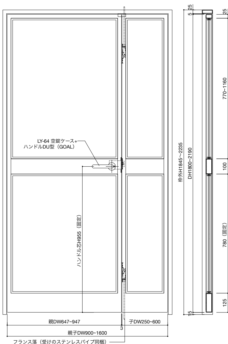
扉裏 立面図 S=1:10
