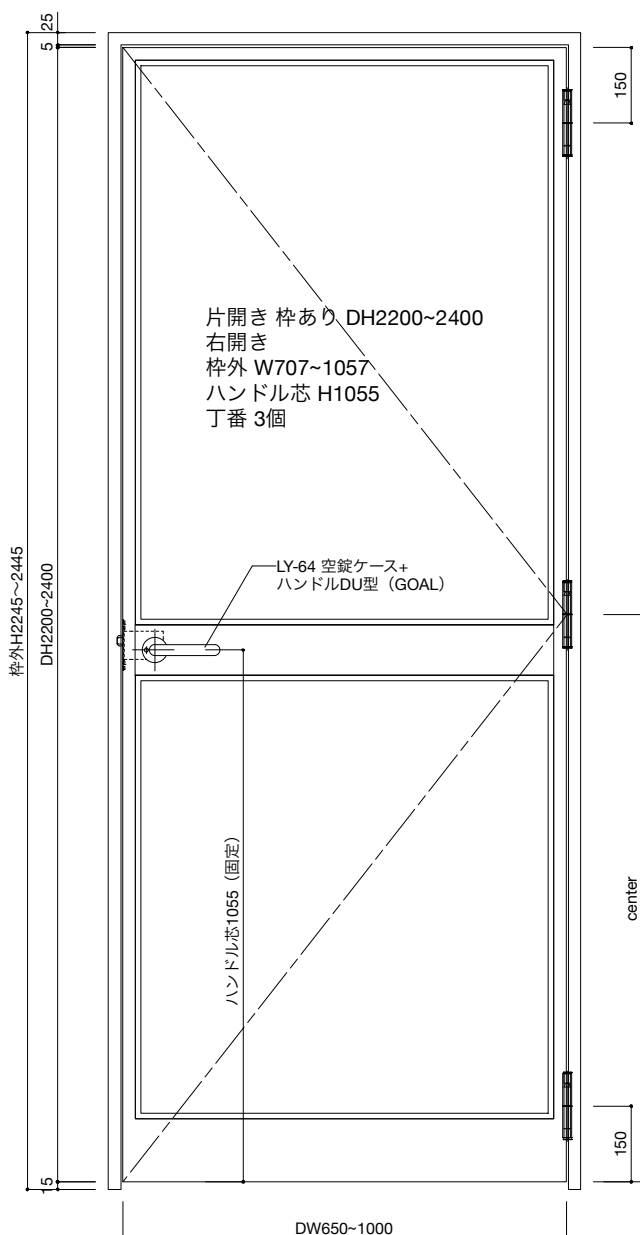
立面図 S=1:10
