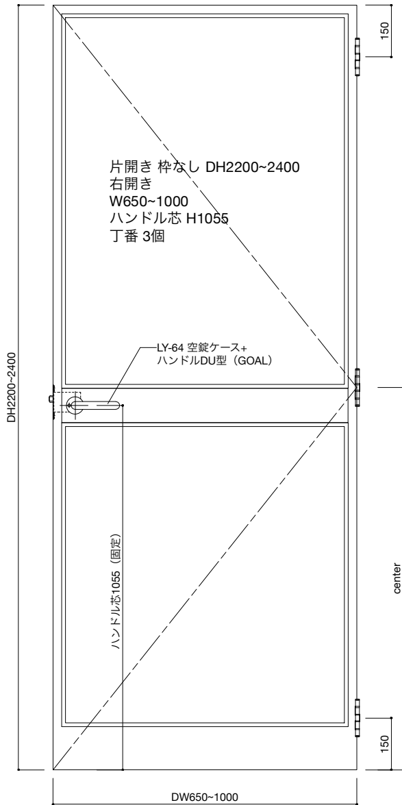
立面図 S=1:10
