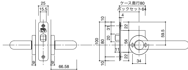
ハンドル詳細図 1/5
