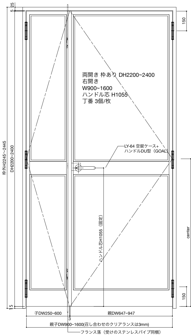
扉表 立面図 S=1:10
