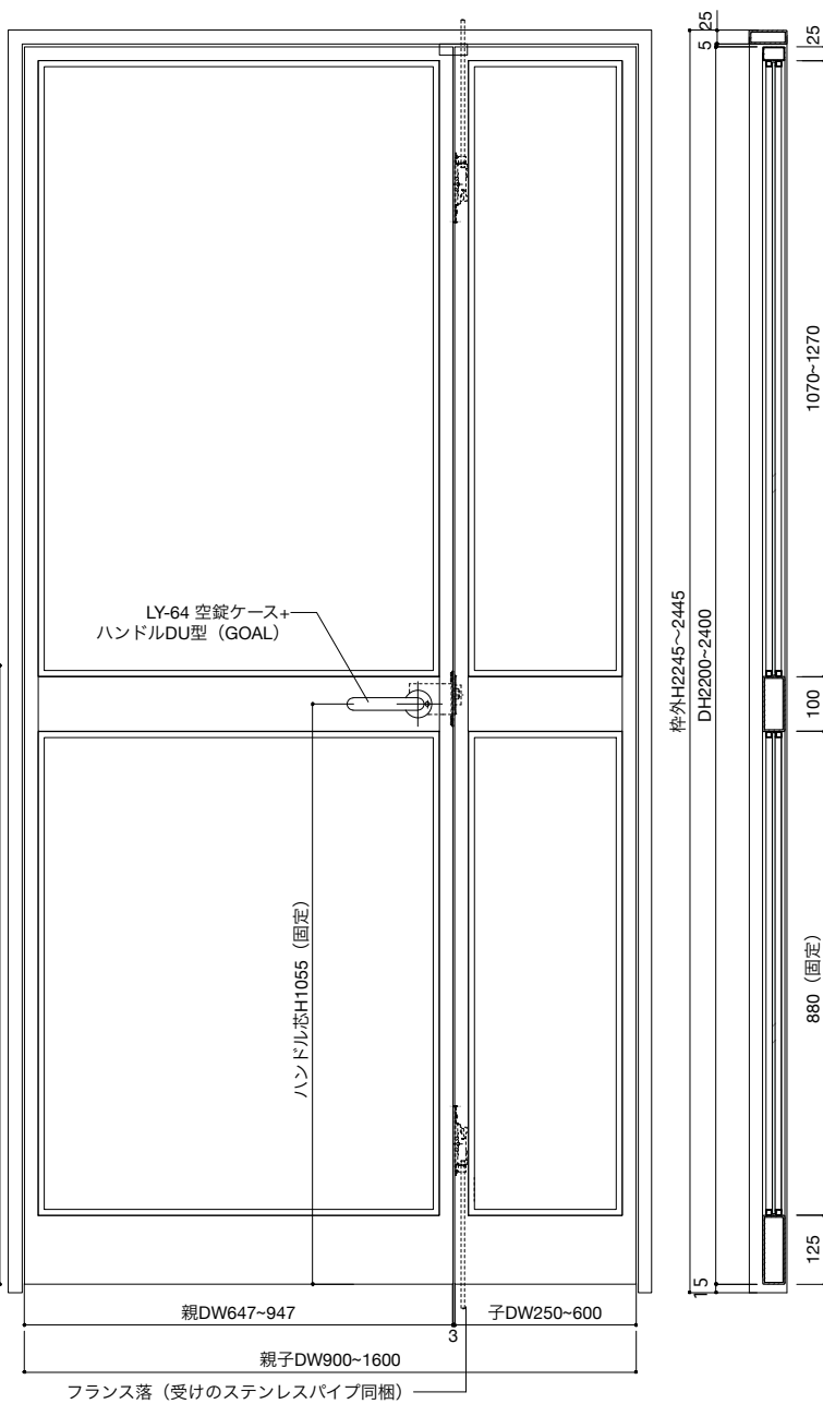
扉裏 立面図 S=1:10
