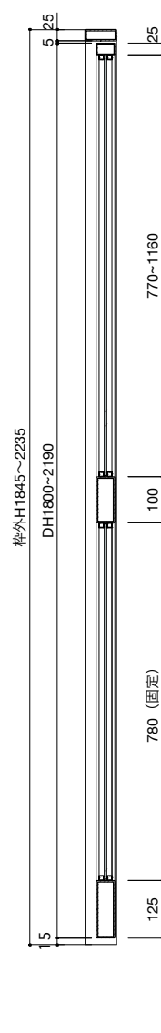
断面図 S=1:10
