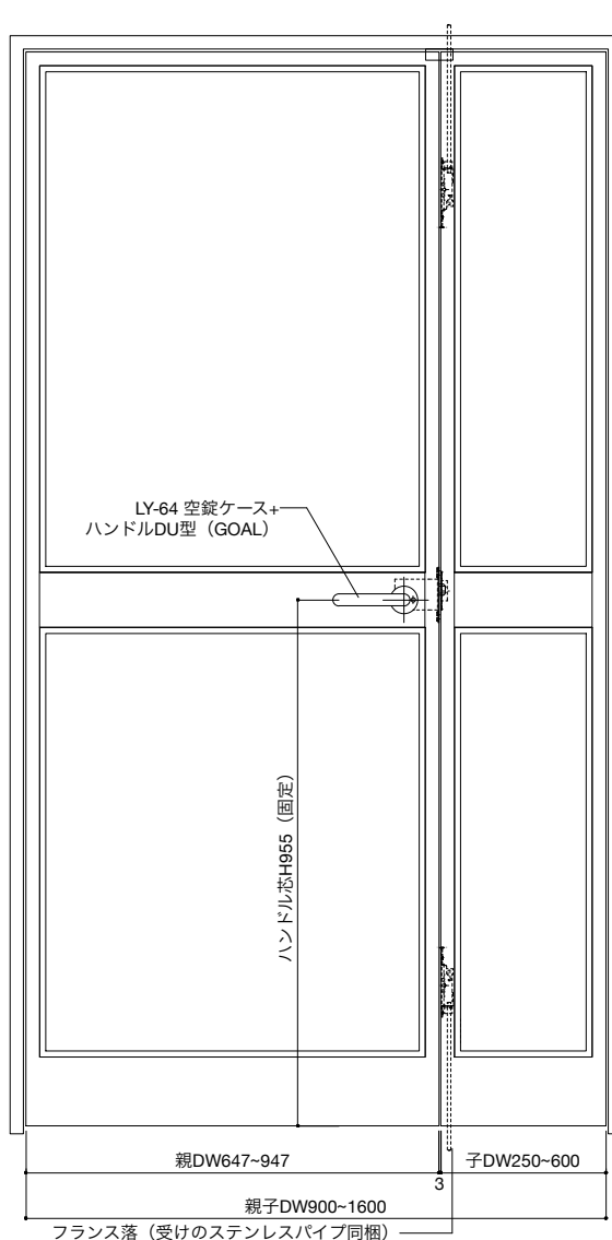
扉裏 立面図 S=1:10
