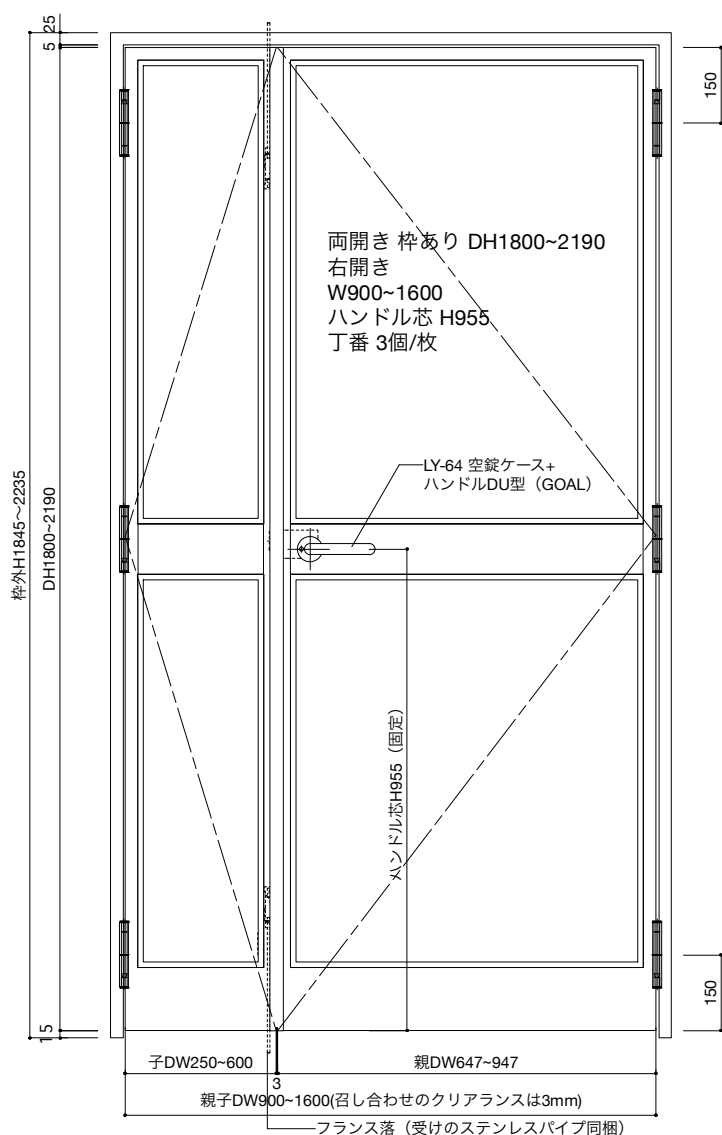
扉表 立面図 S=1:10
