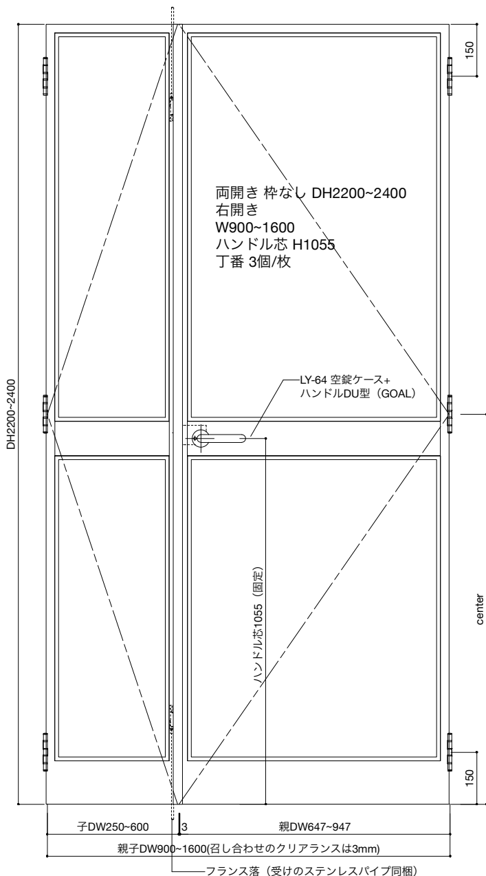
扉表立面図 S=1:10
