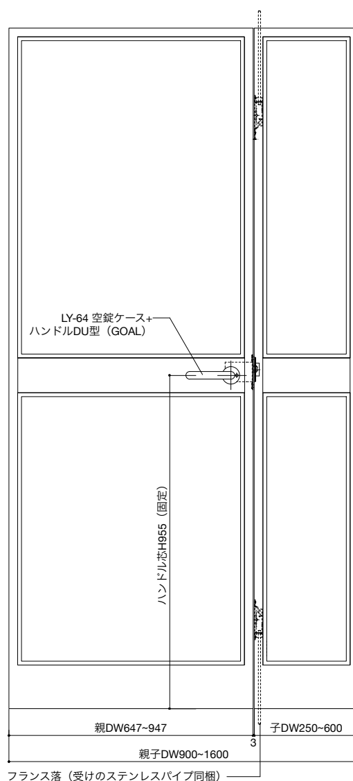
扉裏 立面図 S=1:10
