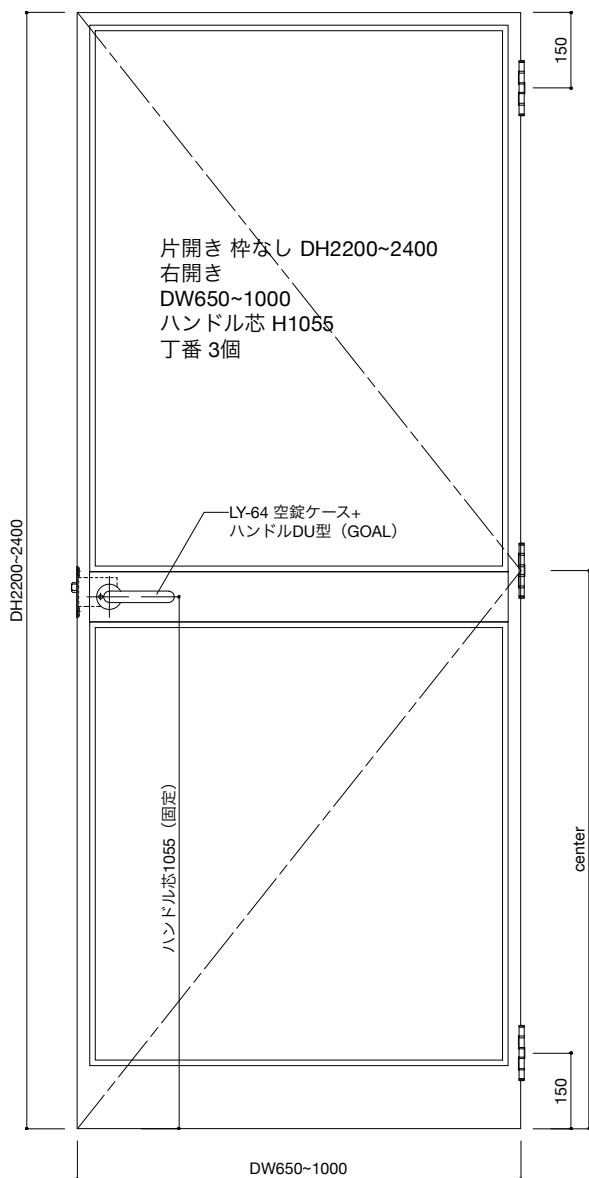
立面図 S=1:10
