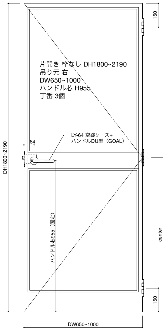
立面図 S=1:10
