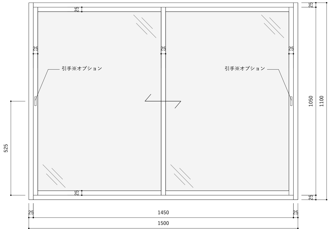
W1500*H900 立面図
