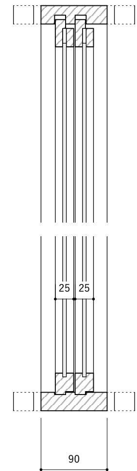
立断面図 S=1:5
