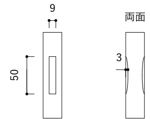
※オプション 引手 握り込み両面 S=1:5
