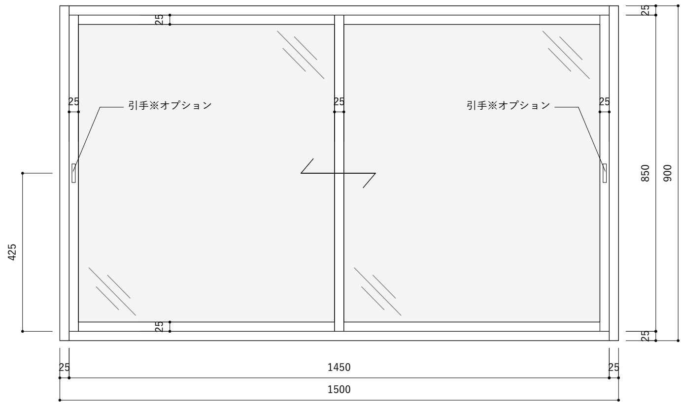
W1500*H900 立面図
