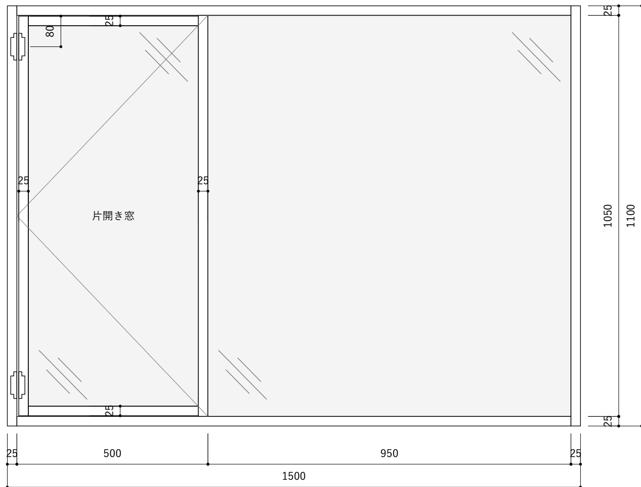
W1500*H1100左タイプ 立面図
