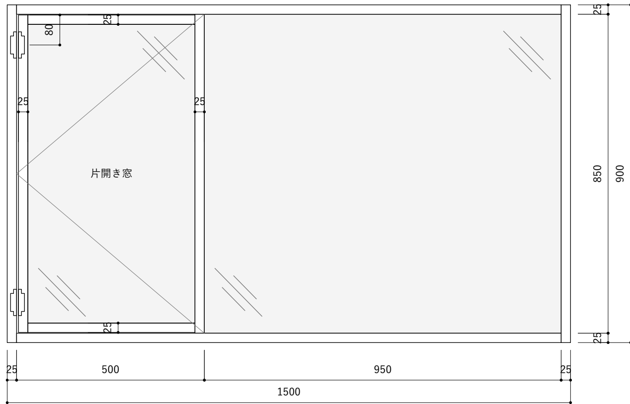
W1500*H900左タイプ 立面図
