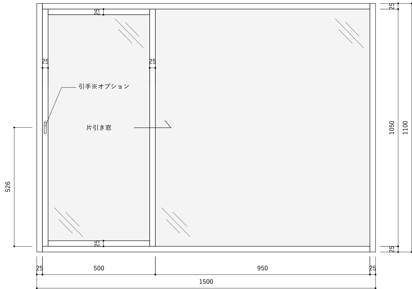
W1500*H1100左タイプ 立面図
