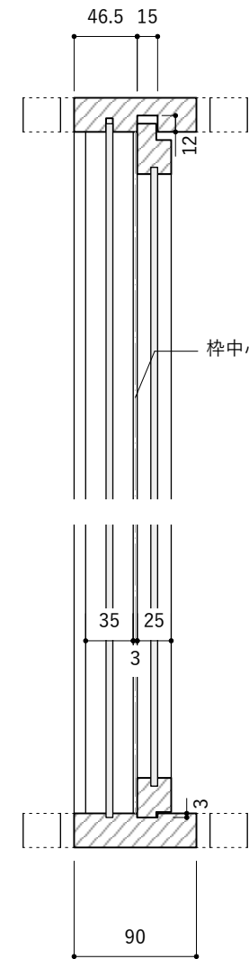
立断面図 S=1:5
