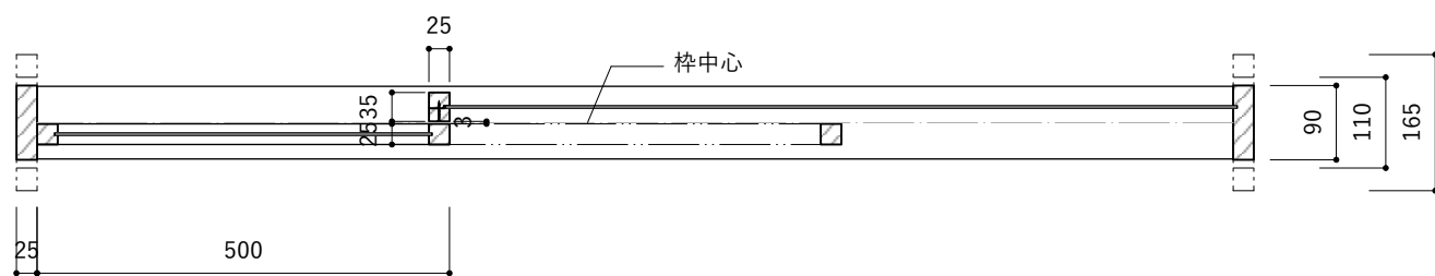
W1500*H1100左タイプ 平断面図
