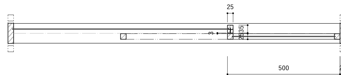
W1500*H900右タイプ 平断面図
