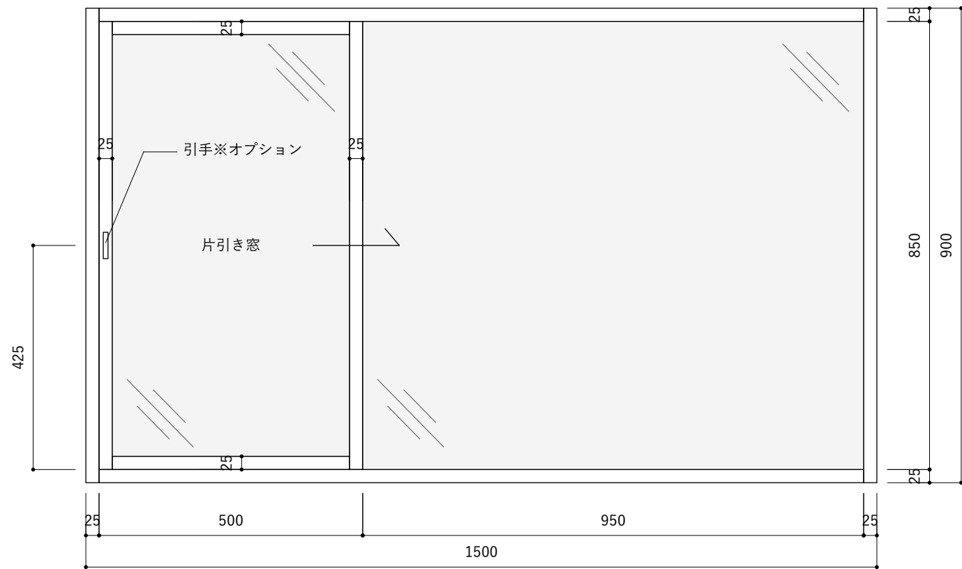
W1500*H900左タイプ 立面図
