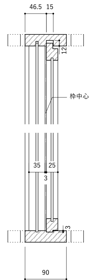
立断面図 S=1:5
