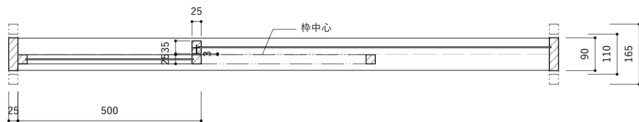
W1500*H900左タイプ 平断面図
