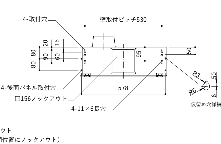
背面取付図
