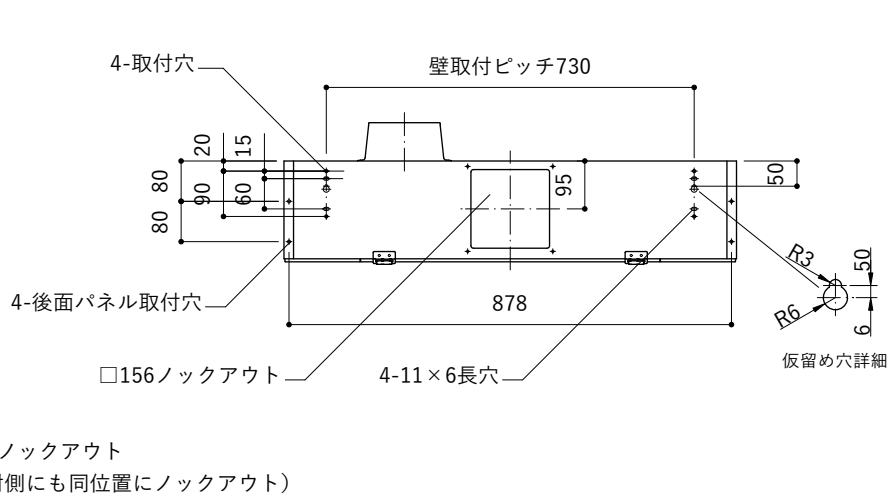
背面取付図
