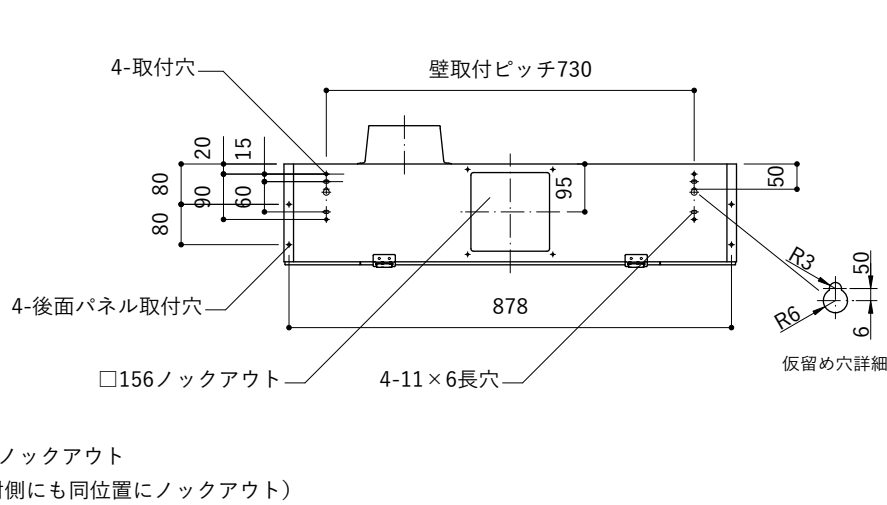
背面取付図
