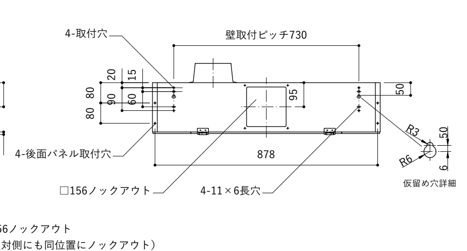
背面取付図
