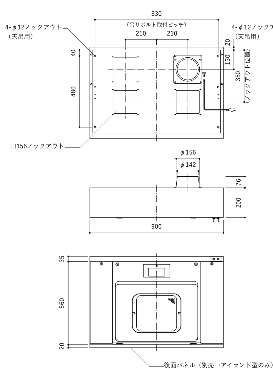
後面パネル取付の場合
