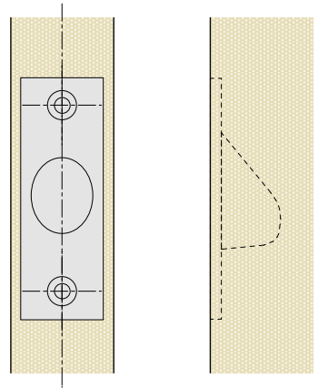
木口手掛け (オプション) S=1:2
