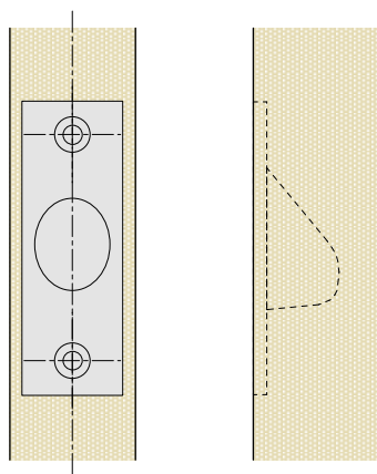
木口手掛け (オプション) S=1:2
