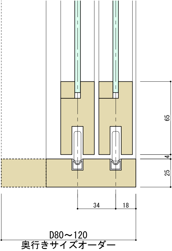
断面詳細図 S=1:2
