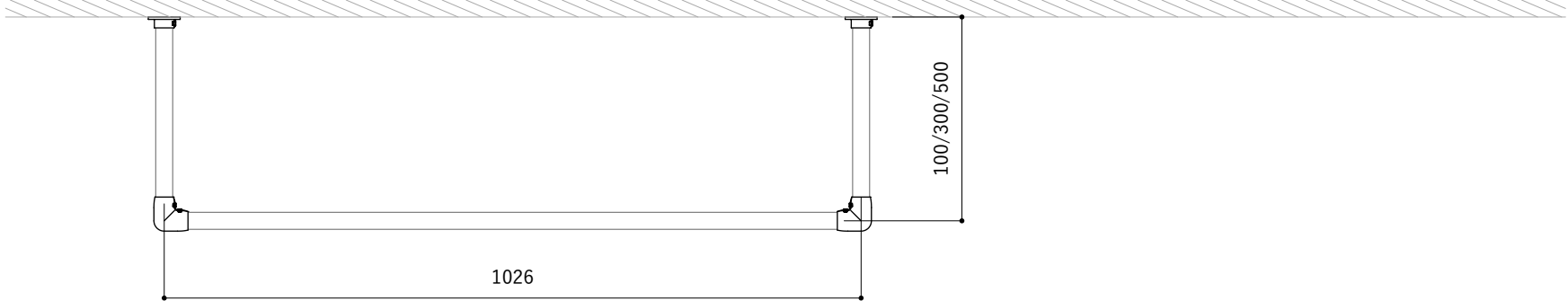
水平パイプ長さ(L)1000
