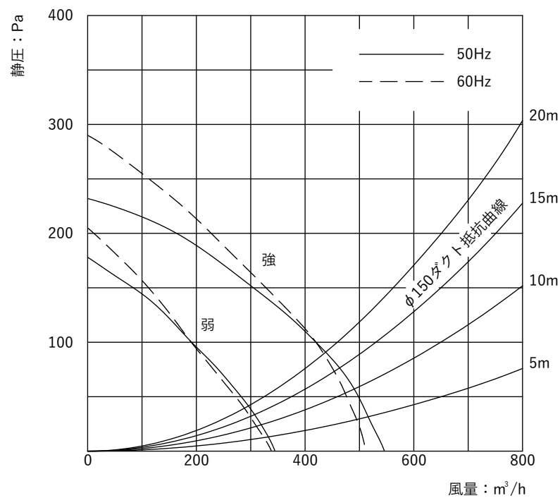
□静圧 - 風量曲線
