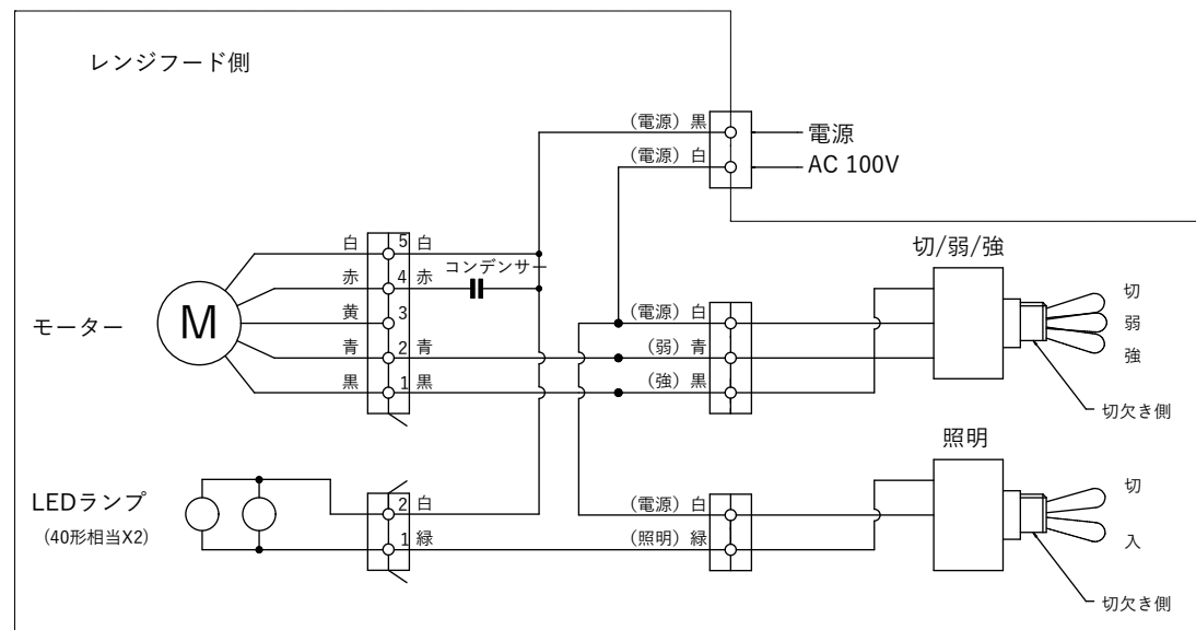
結線図
