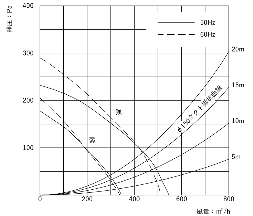
□静圧 - 風量曲線
