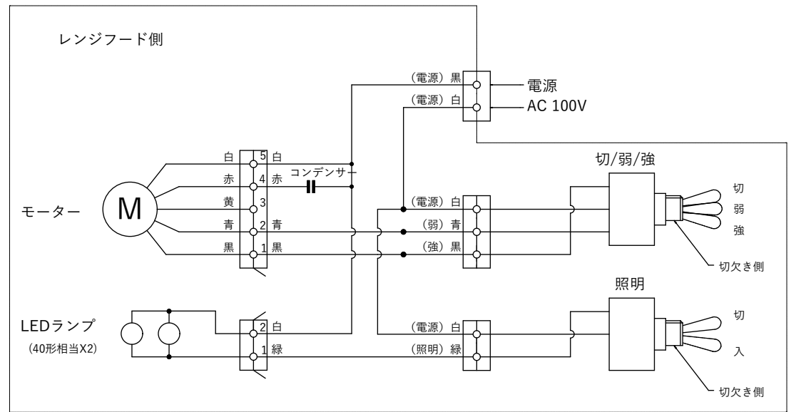
結線図
