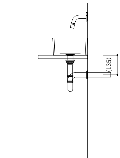
【側面図・Pトラップ】
