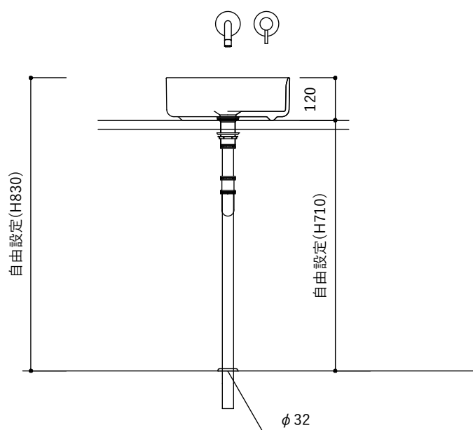
【正面図・Sトラップ】
