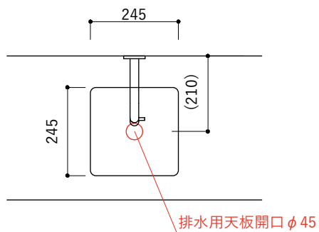
【正面図・Sトラップ】
