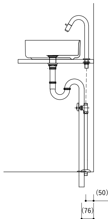
【側面図・Pトラップ】
