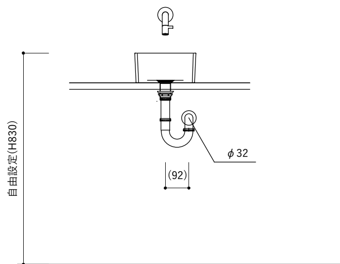
【正面図・Pトラップ】
