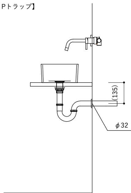
【側面図・Pトラップ】
