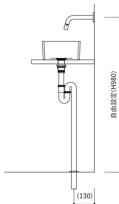
【側面図・Sトラップ】
