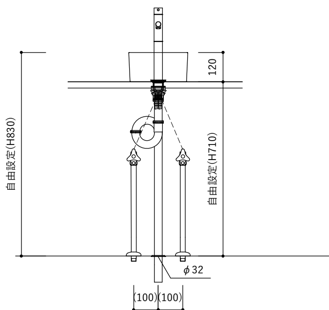
【正面図・Pトラップ】
