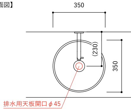
【正面図・Sトラップ】
