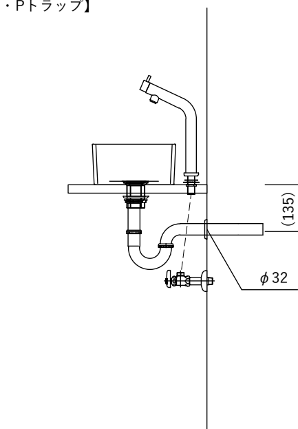
【側面図・Pトラップ o 】
