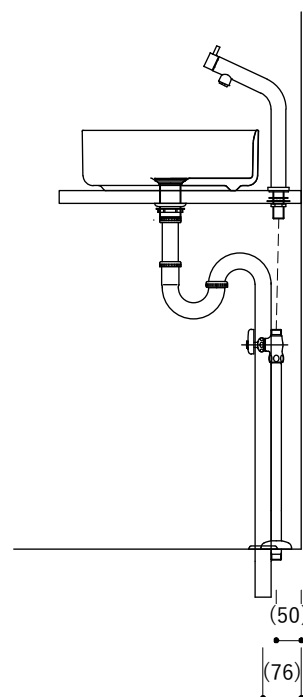
【側面図・Sトラップ】
