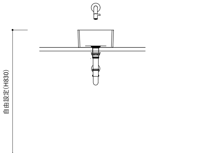
【正面図・Pトラップ】
