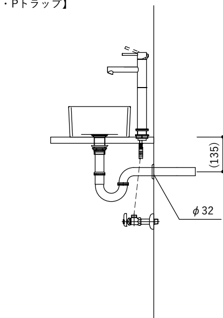
【側面図・Pトラップ】
