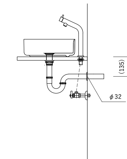
【側面図・Pトラップ】
