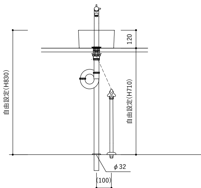
【正面図・Pトラップ】
