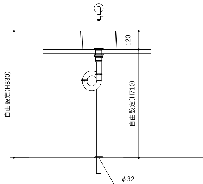
【正面図・Sトラップ】
