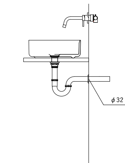
【側面図・Pトラップ】
