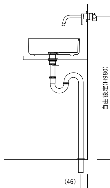
【側面図・Sトラップ】
