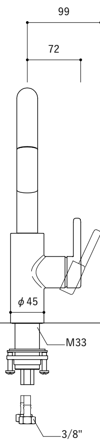
正面図
