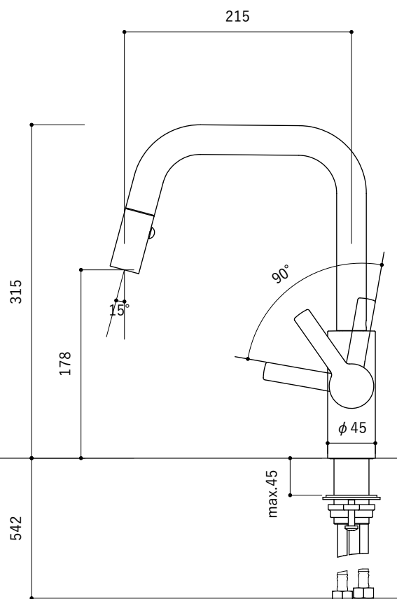
右側面図
