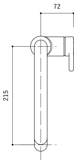
平面図
