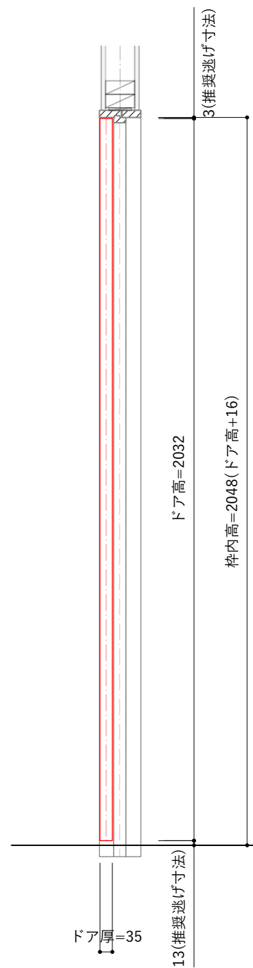
立面図 S=1 : 15
