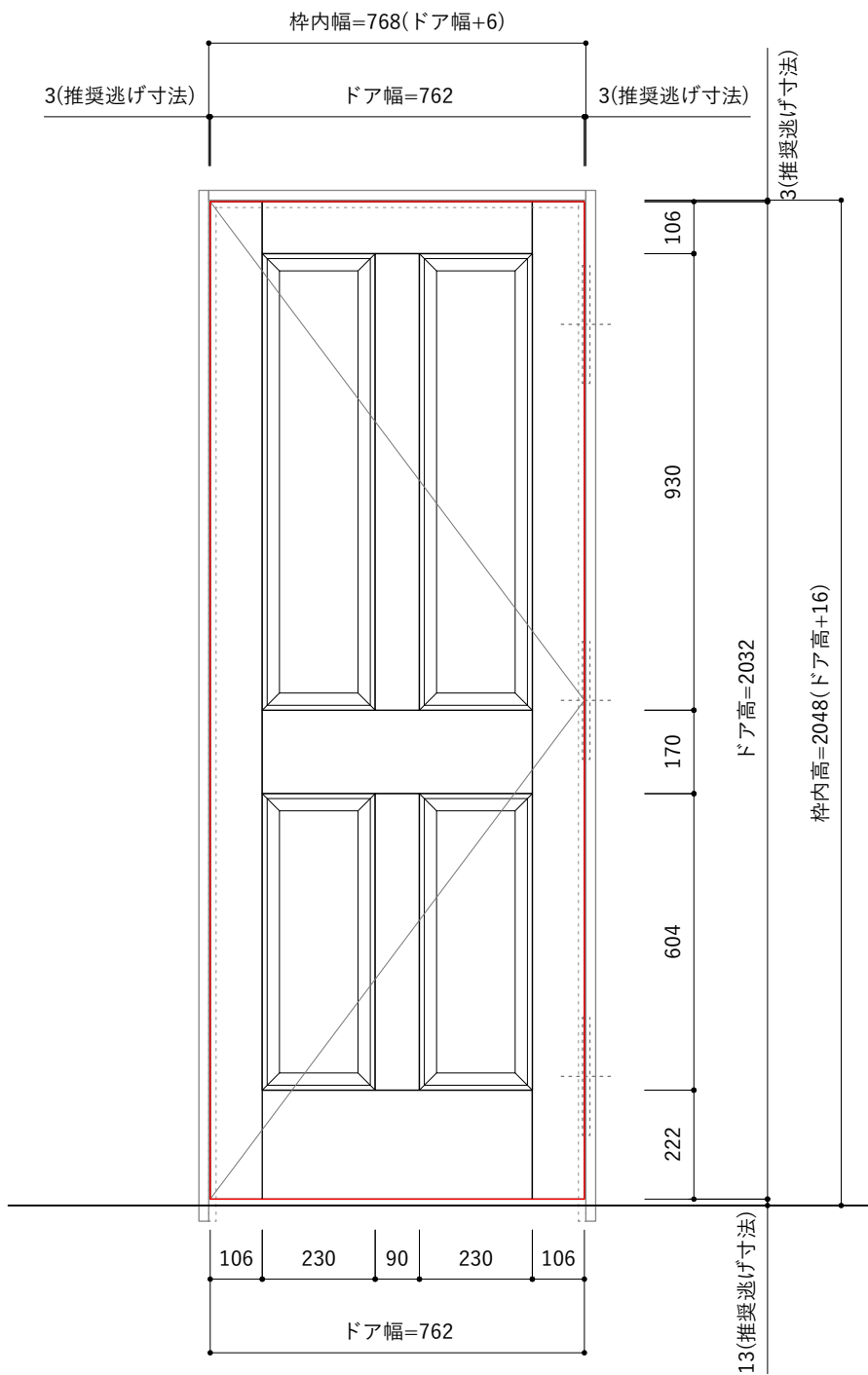
立面図 S=1 : 15
