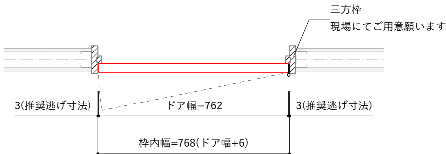
平面図 S=1 : 15
