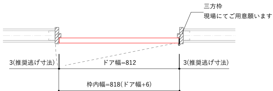
平面図 S=1 : 15
