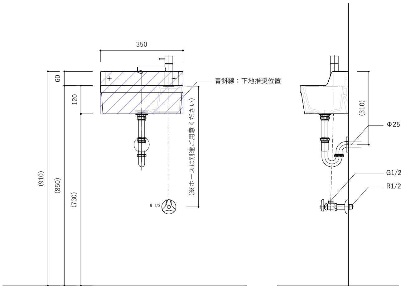
正面図
