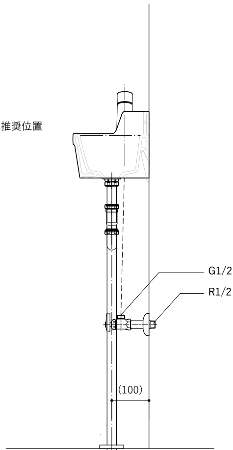
断面図
