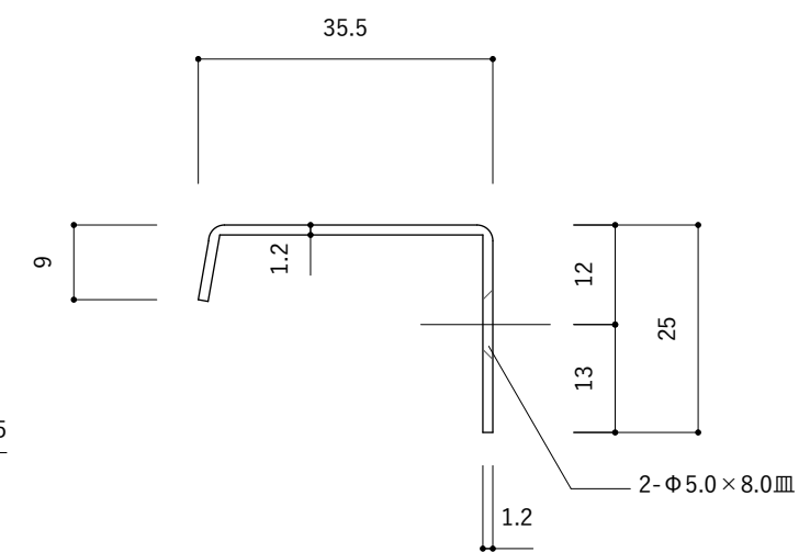
側面図(共通)
