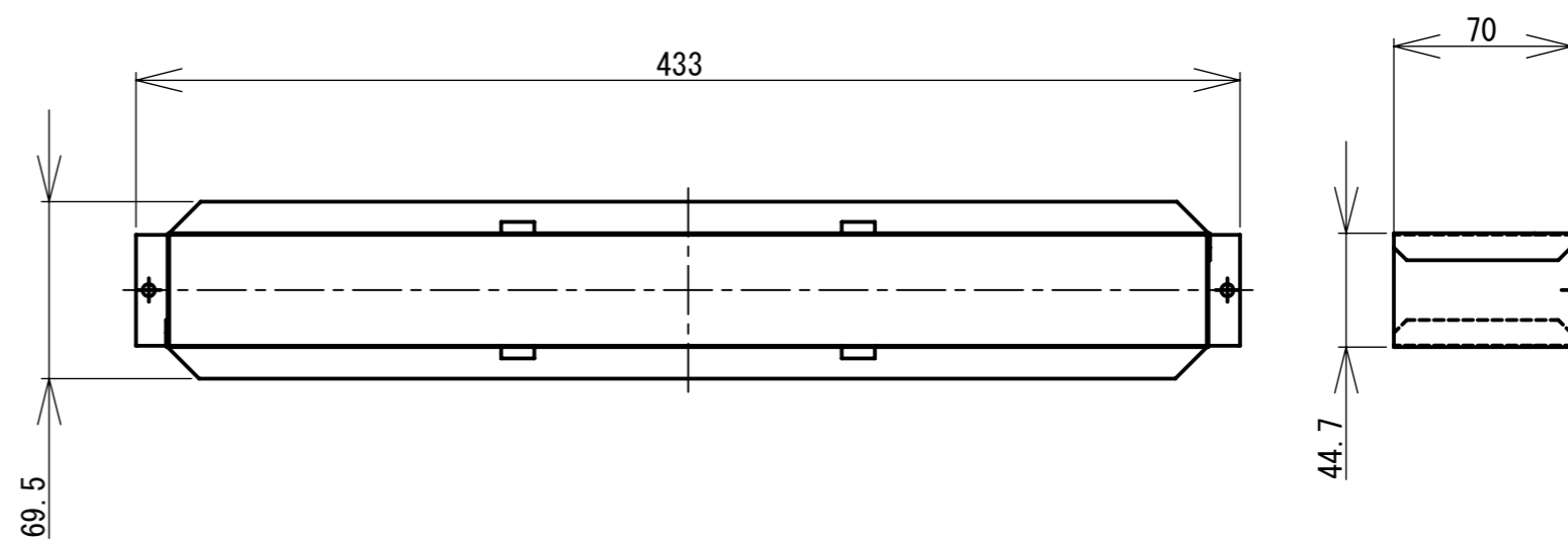
中間排気筒
