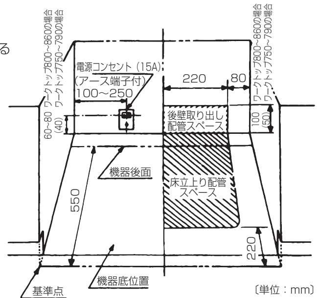
ガス配管・電源コンセント取り出し位置図
