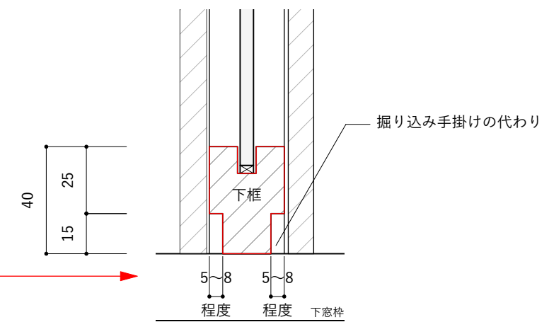
部分縦断面図 S=1:2
