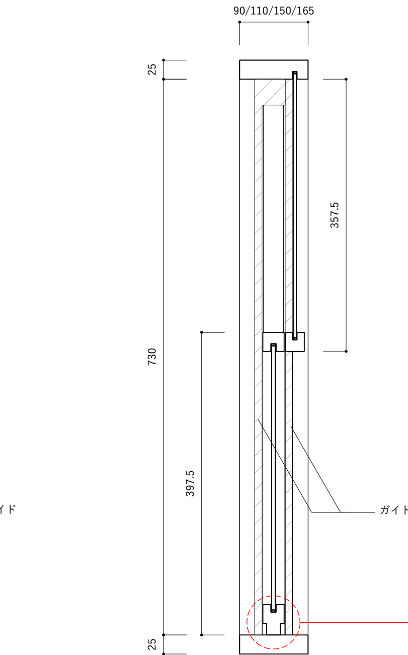
縦断面図 S=1:15
