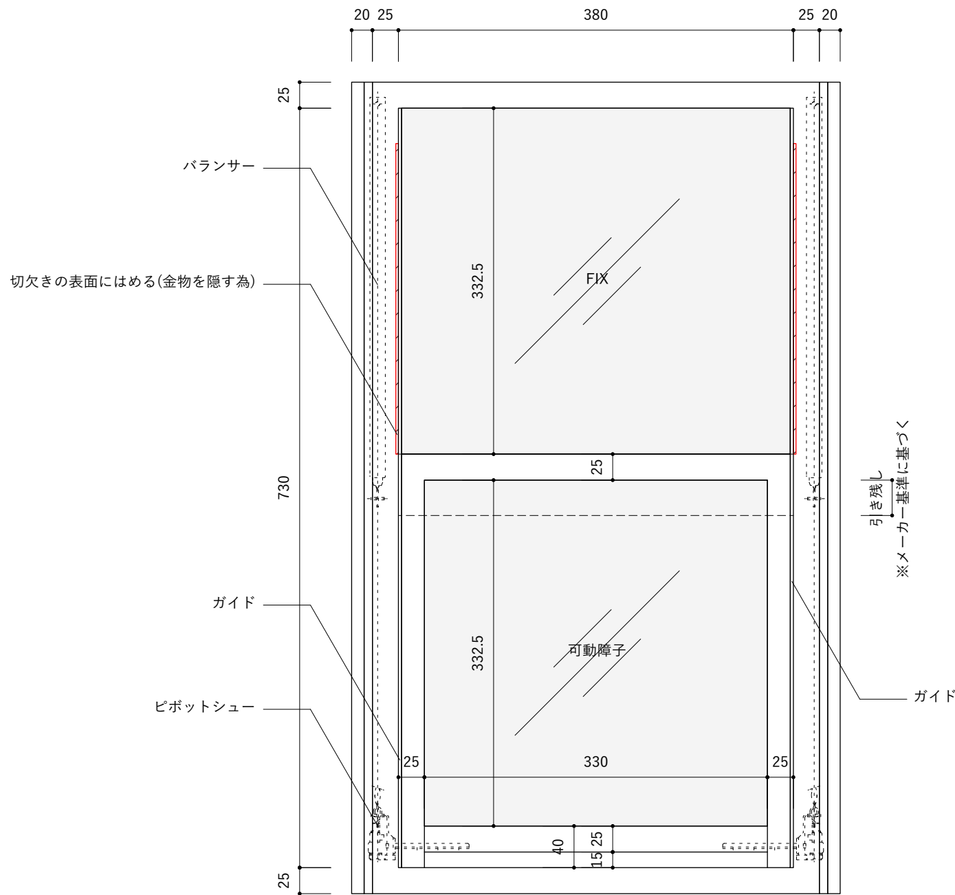
正面図 S=1:15
