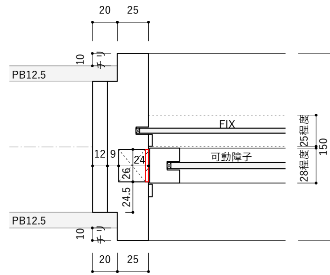
部分横断面図 150幅 S=1:3
