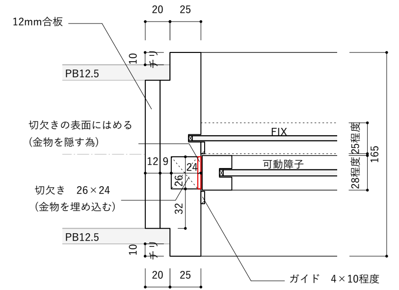
部分横断面図 165幅 S=1:3
