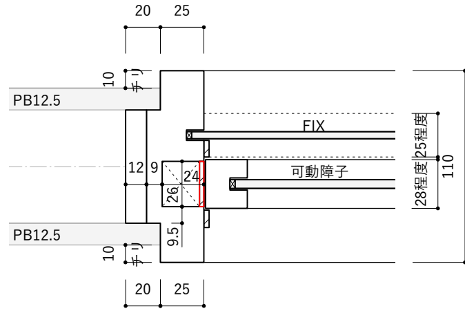
部分横断面図 110幅 S=1:3
