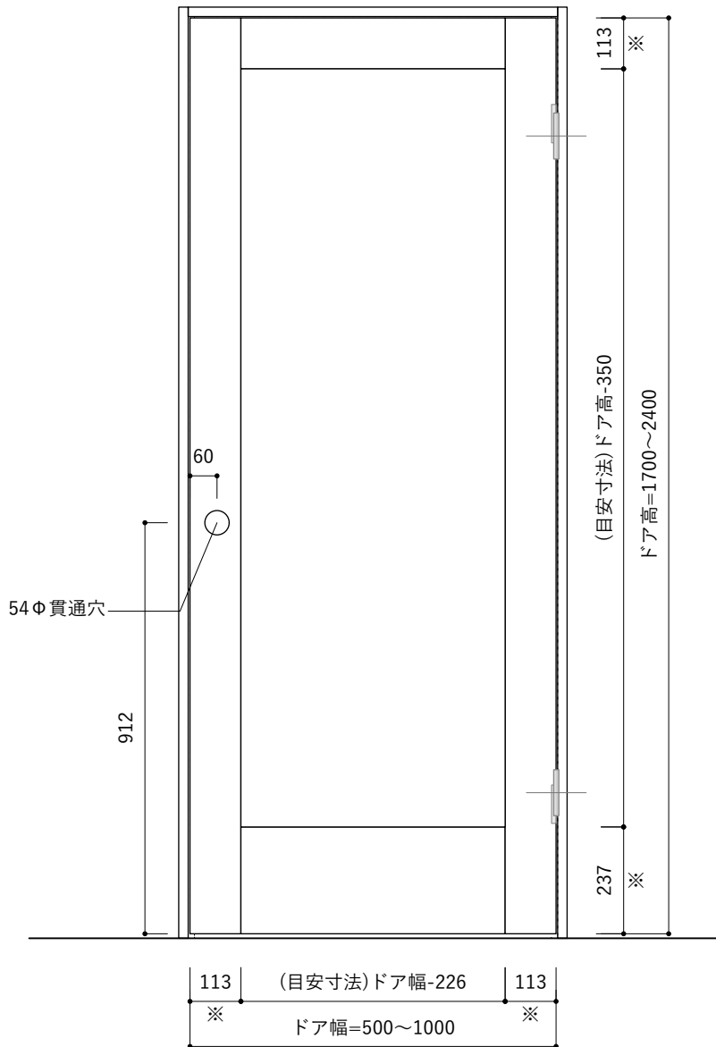
立面図 S=1 : 15
