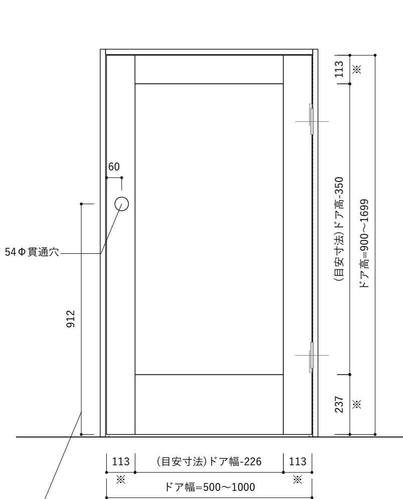
立面図 S=1 : 15
