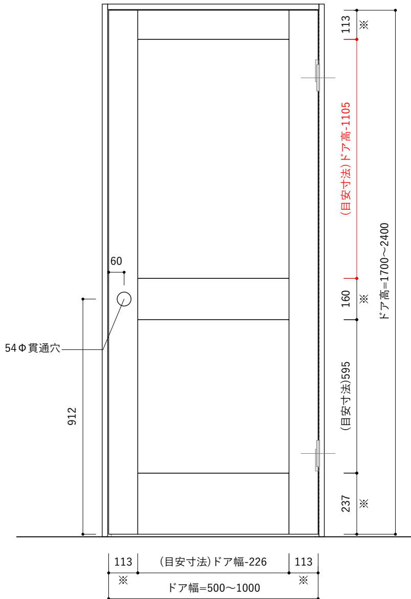
立面図 S=1 : 15
