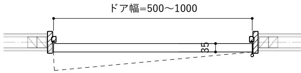
平面図 S=1 : 15
