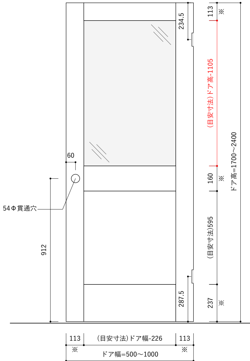
立面図 S=1 : 15
