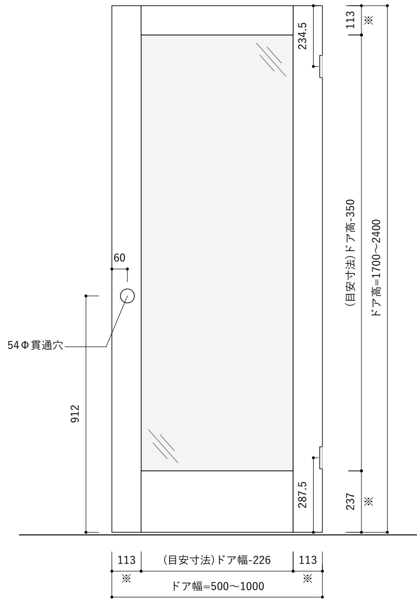
立面図 S=1 : 15
