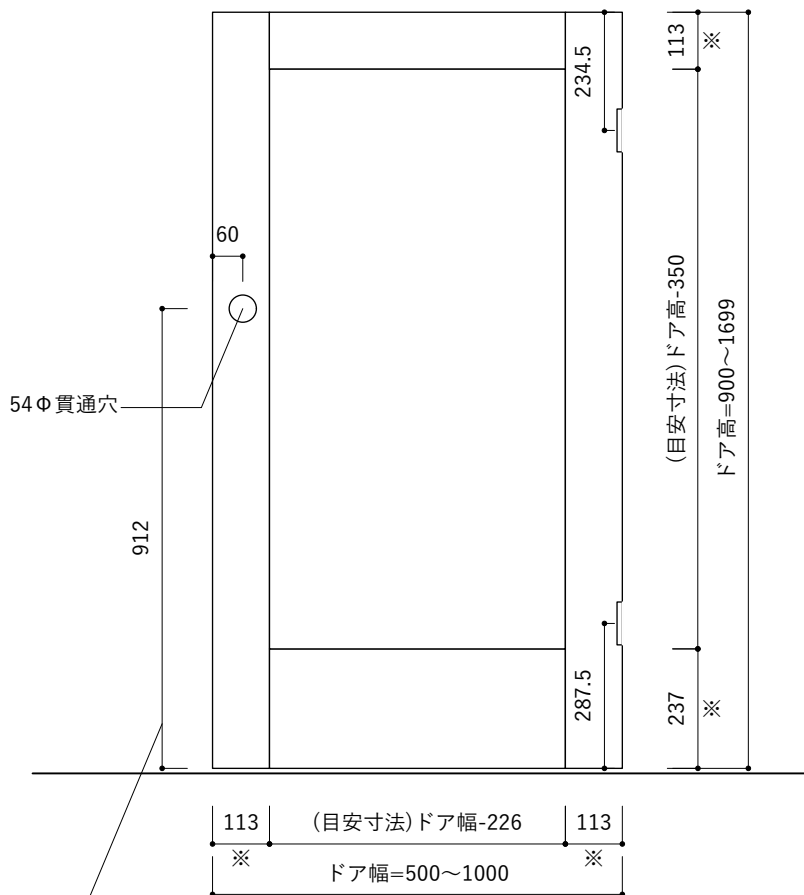
立面図 S=1 : 15
