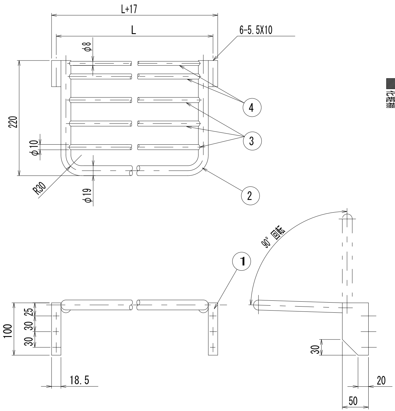
標準パイプ棚寸法 L-300m/m
