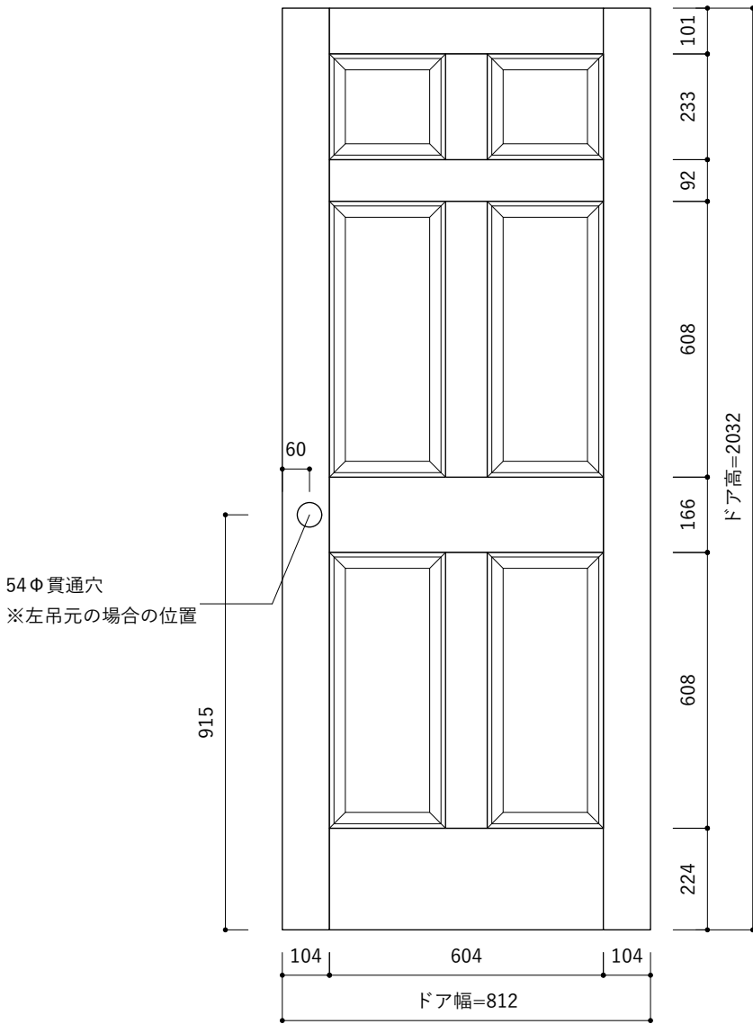
立面図 S=1 : 15
