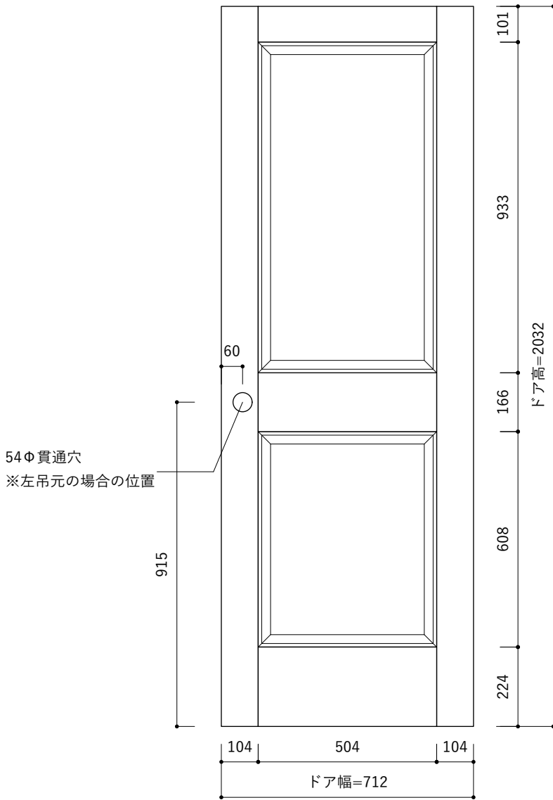
立面図 S=1 : 15
