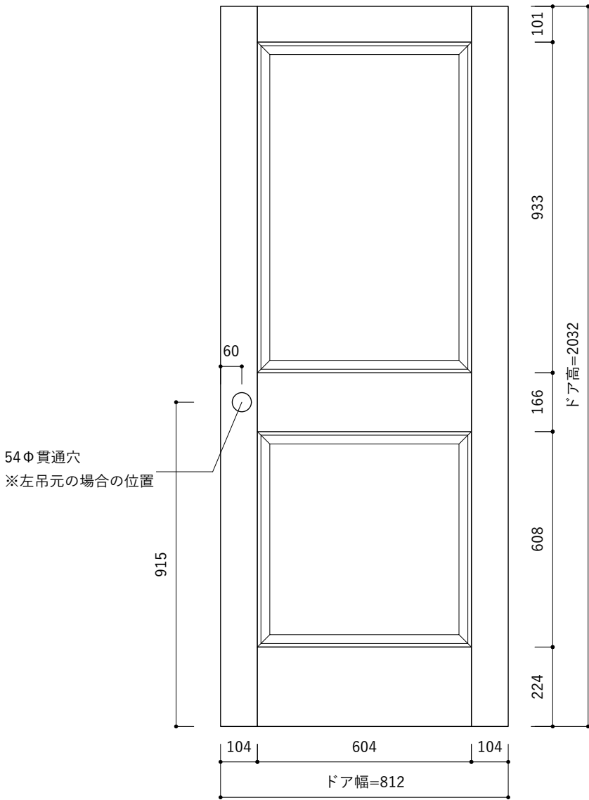
立面図 S=1 : 15
