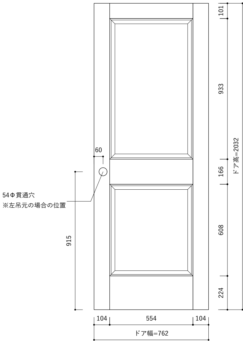
立面図 S=1 : 15
