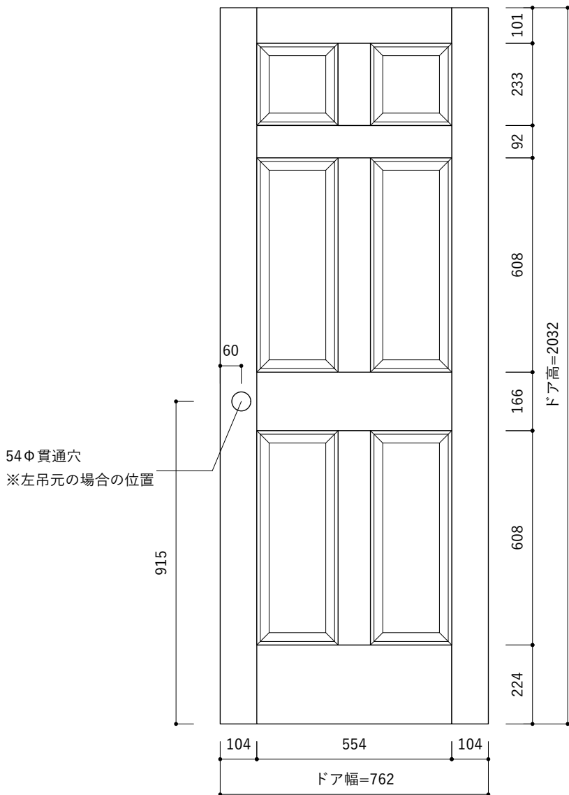
立面図 S=1 : 15
