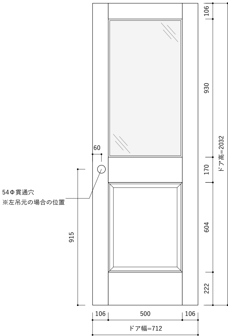
立面図 S=1 : 15
