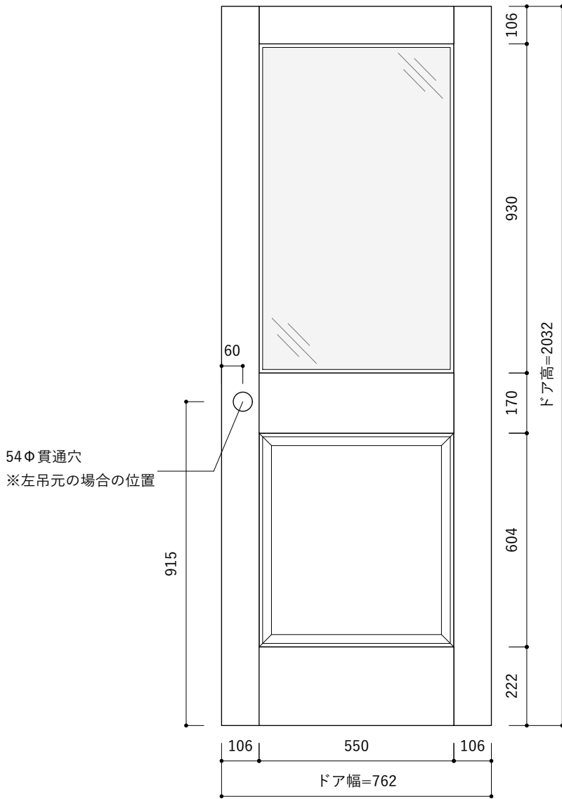
立面図 S=1 : 15
