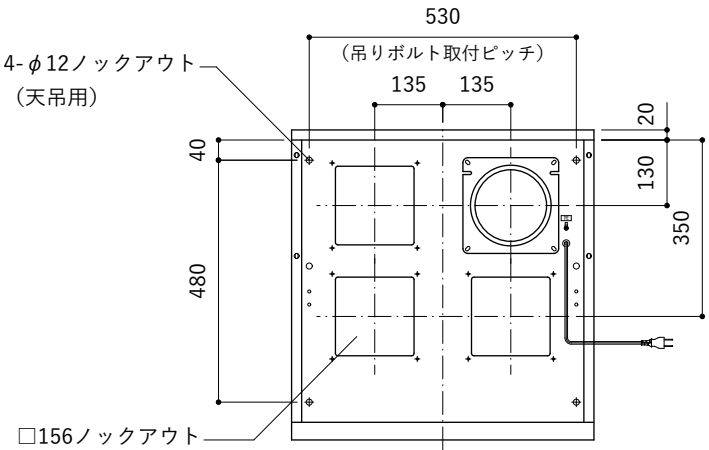
後面パネル取付の場合
