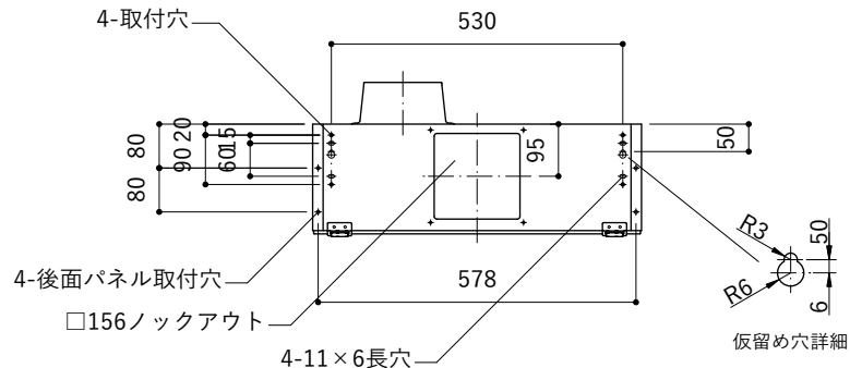
背面取付図
