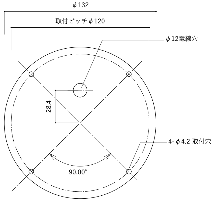
【取付面 寸法図】
