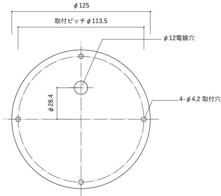
【取付面 寸法図】
